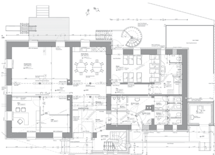
Grundriss des Erdgeschoßes mit der geplanten Kinderkrippe (Pläne Architekturbüro Martin)
